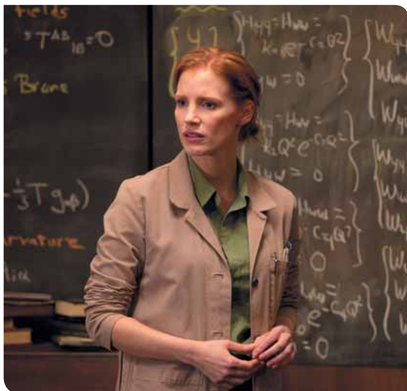
Существование пятого измерения из фильма «Интерстеллар» (2014) предсказывают физические расчеты.
